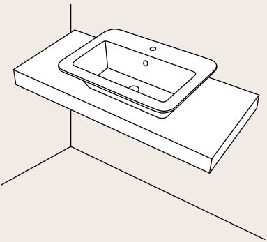
installazione da appoggio su piano on top installation 64 x 49 x h13 - OPLA64R
