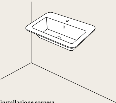
installazione sospesa wall-hung installation 64 x 49 x h13 - OPLA64R
