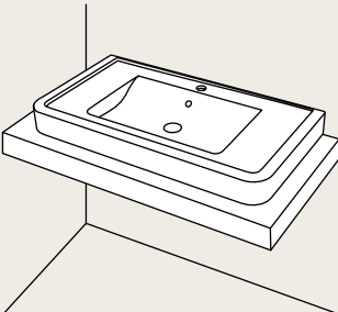
installazione da appoggio su piano on top installation 100 x 56 x h11 - OPC100
