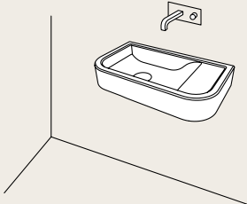
installazione sospesa con rubinetto a parete suspended installation with taps on wall 45 x 25 x h8 - OPLA45
