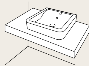
installazione da appoggio su piano on top installation 52 x 52 x h11 - OPLA52
