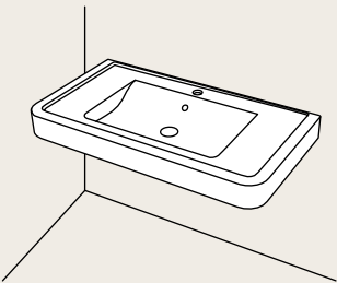
installazione sospesa wall-hung installation 100 x 56 x h11 - OPC100
