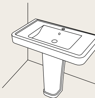
installazione su colonna on pedestal installation 100 x 56 x h11 - OPC100 + OPCOL
