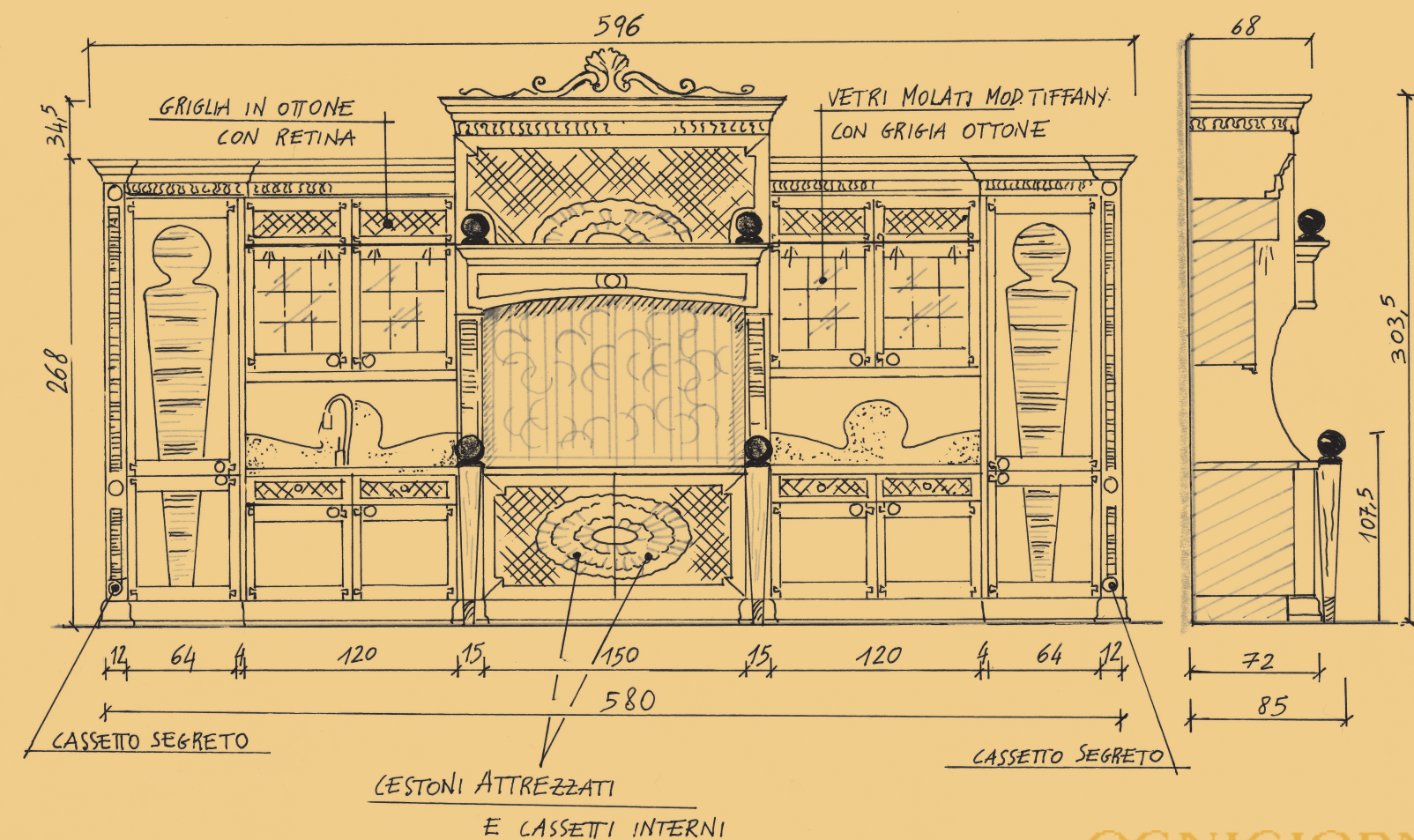
Cucina MAJESTIC – PROGETTAZIONE E VALORI DIMENSIONALI MAJESTIC kitchen – DESIGN AND DIMENSIONAL VALUES
