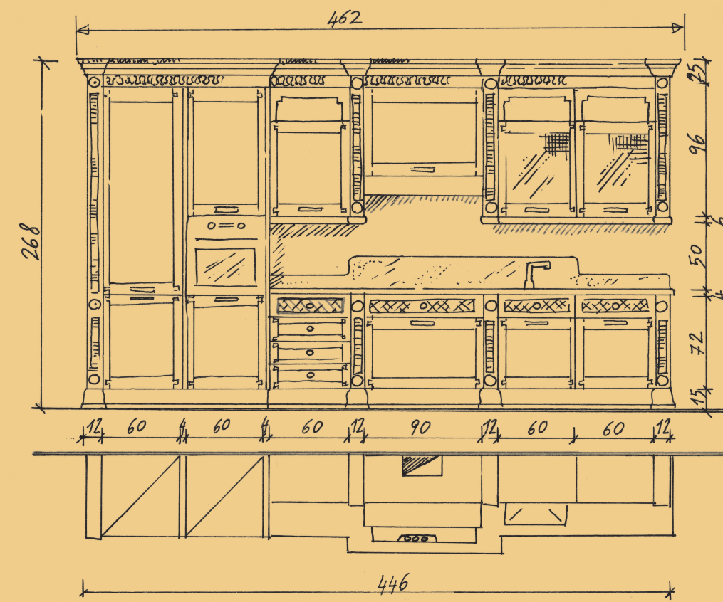
Cucina MAJESTIC – PROGETTAZIONE E VALORI DIMENSIONALI MAJESTIC kitchen – DESIGN AND DIMENSIONAL VALUES
